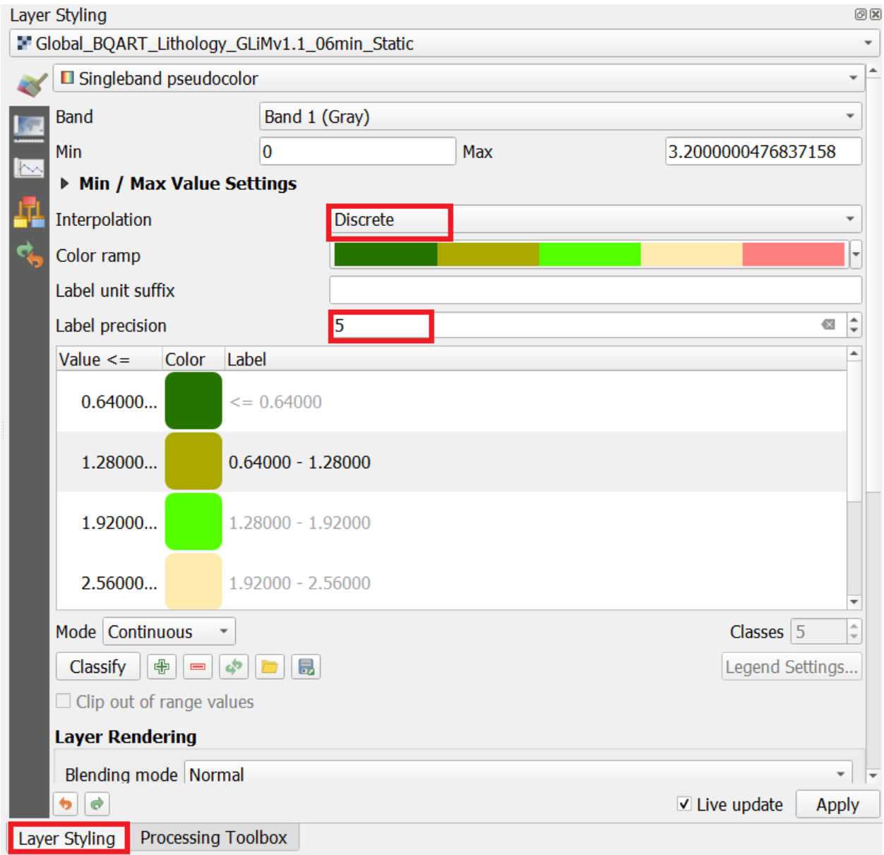
Fig. 2: Layer Styling
